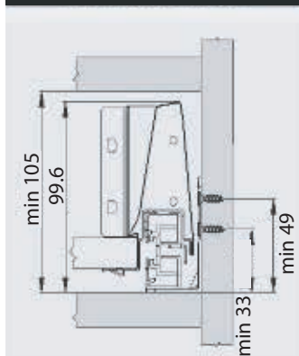
Perforación para panel de frente
