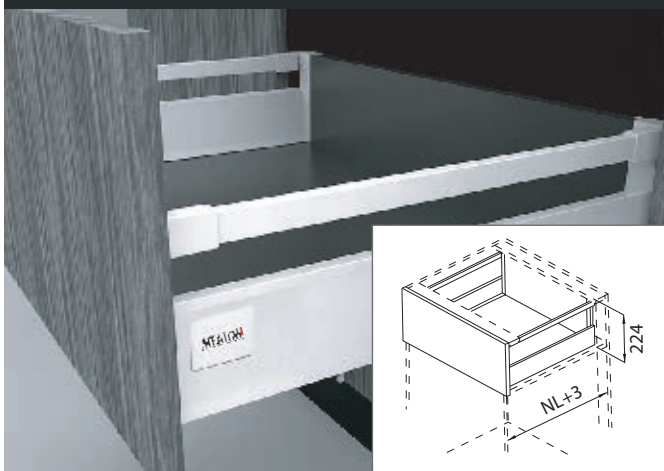
Espacio de cajón
