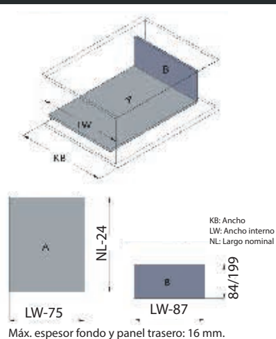
Medidas de corte para panel trasero
