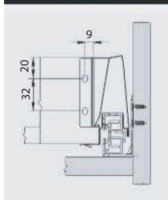
Instalación de correderas
