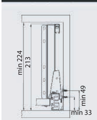
Perforación para panel de frente
