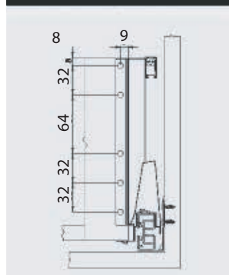
Medidas de corte para panel trasero
