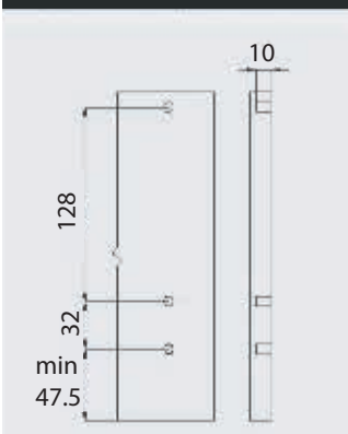
Medidas de corte para panel trasero
