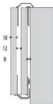
Puerta 18 mm
