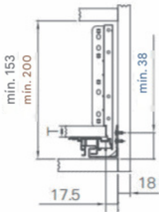
3. Espacio necesario dentro del gabinete
