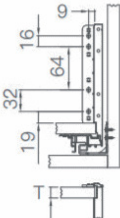
Dimensiones de instalación posterior
