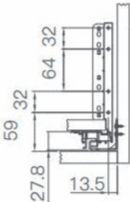
Superposición del panel frontal (FA)
